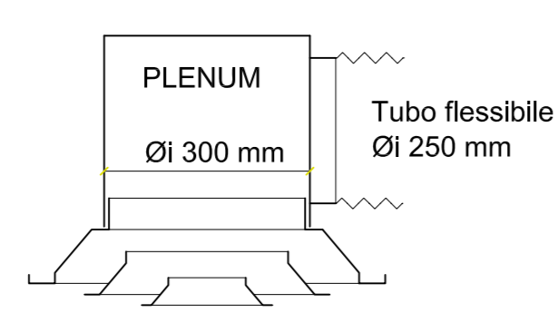
PARTICOLARE BOCCHETTE
