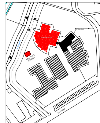
PLANIMETRIA GENERALE scala 1:1000
